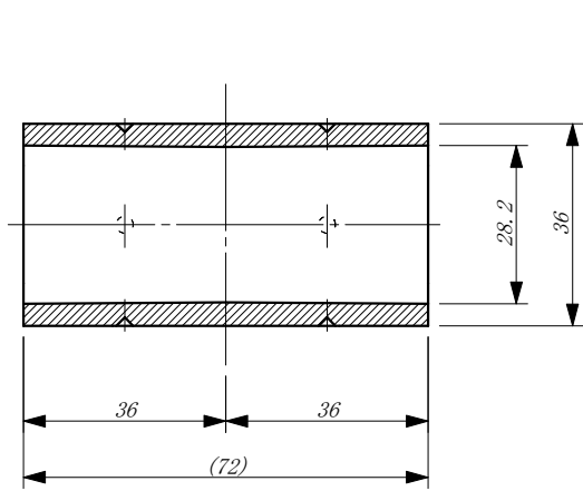
A-A断面
