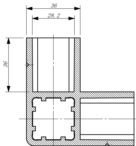
B-B断面
