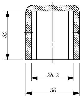
A-A断面
