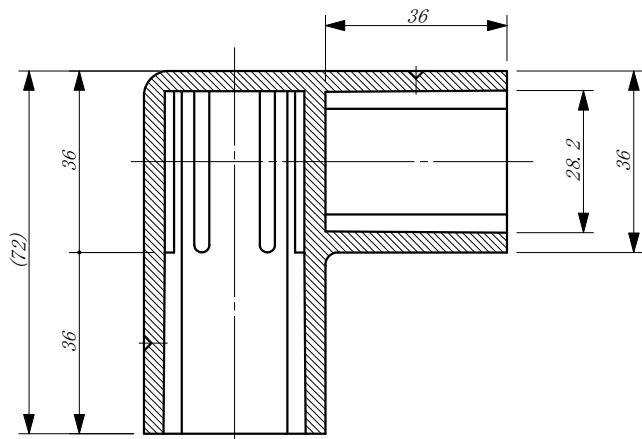
A-A断面
