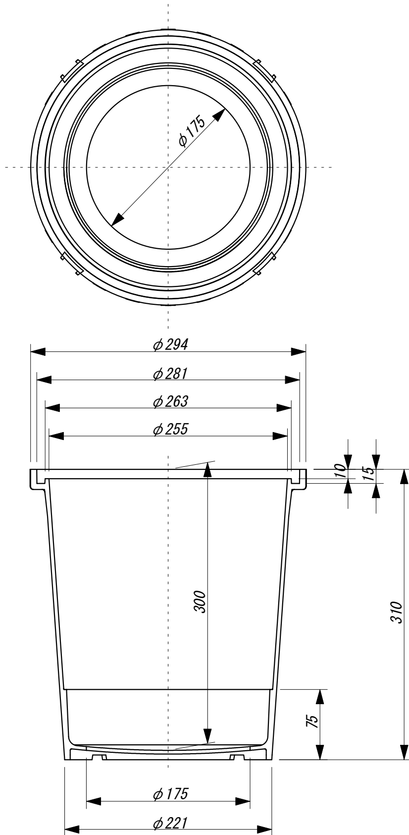
図名 ポリプロピレン製 雨水浸透ます(底穴タイプ) 250型-300H 寸法図
