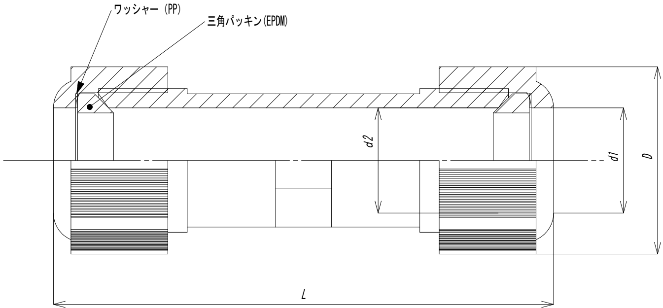
断面図 A-A
