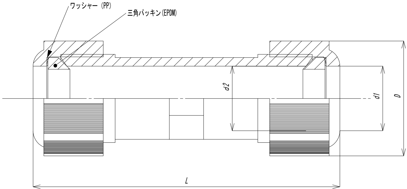
断面図 A-A
